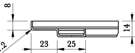
细节 A 比例 1:2
