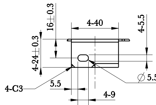
细节 A 比例 1:2 ratio 1:2
