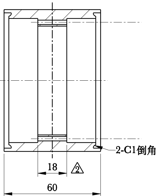
截面B-B
