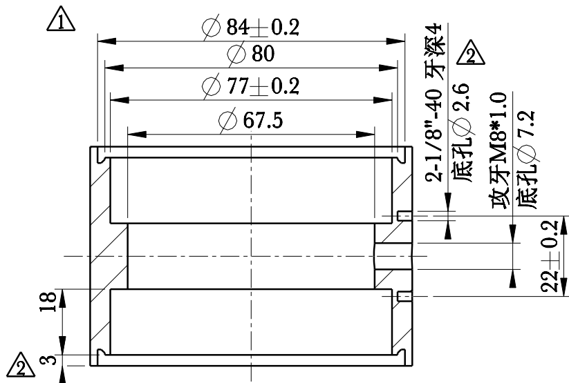
截面A-A
