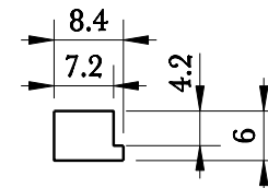
铝挤截面 AL section
