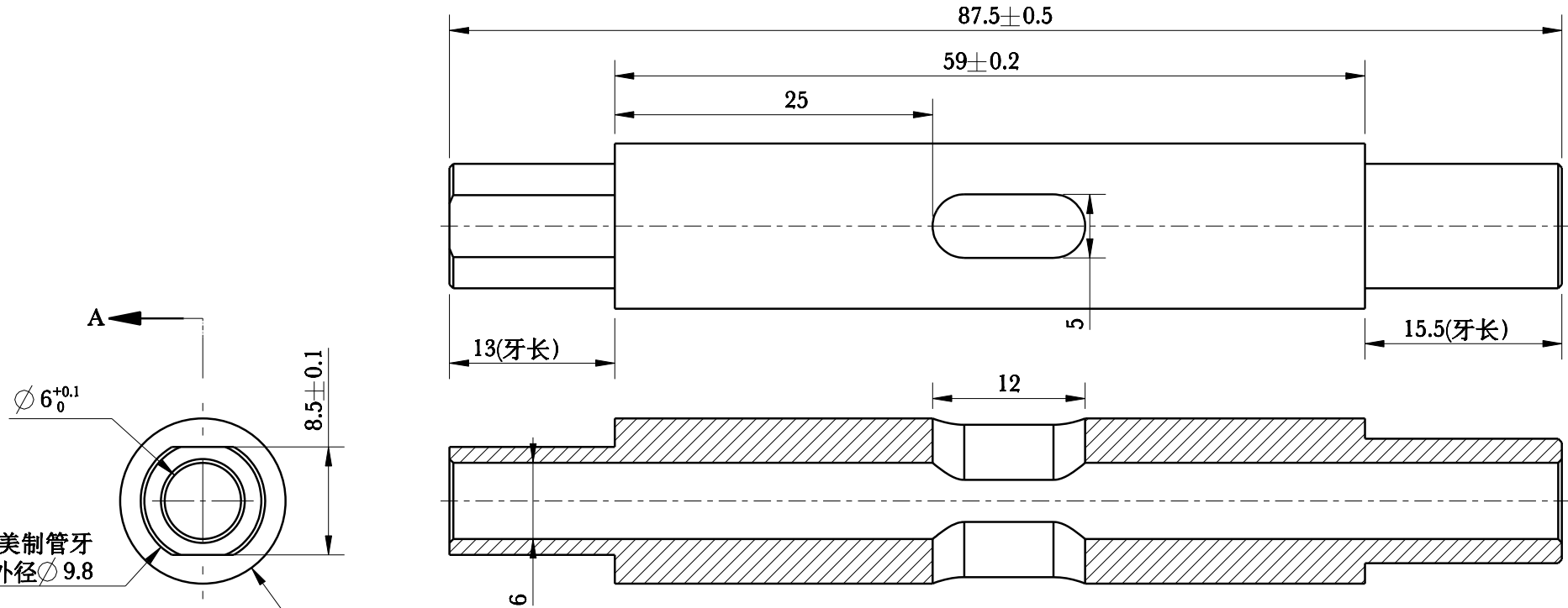
截面 A-A
