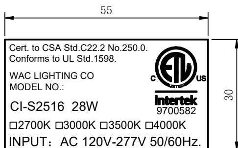
CI-MT-S2516-KIT-1
