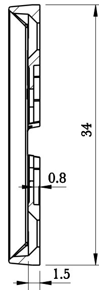
截面 B-B
