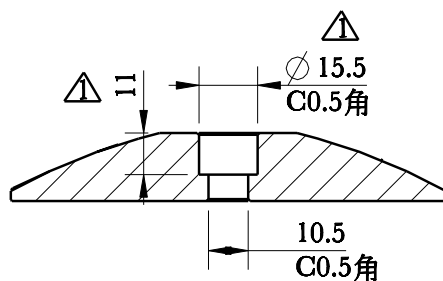
截面 A-A
