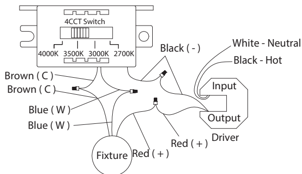
Fig. 4 Wiring
