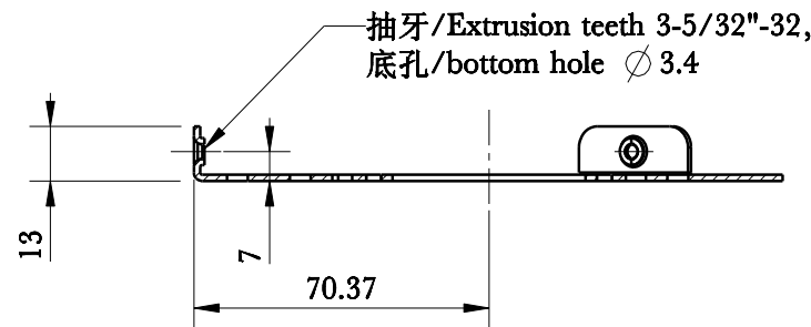
截面 A-A
