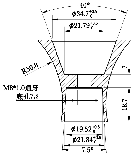
截面 A-A
