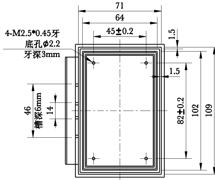
截面 A-A
