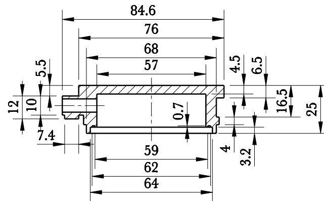
截面 A-A
